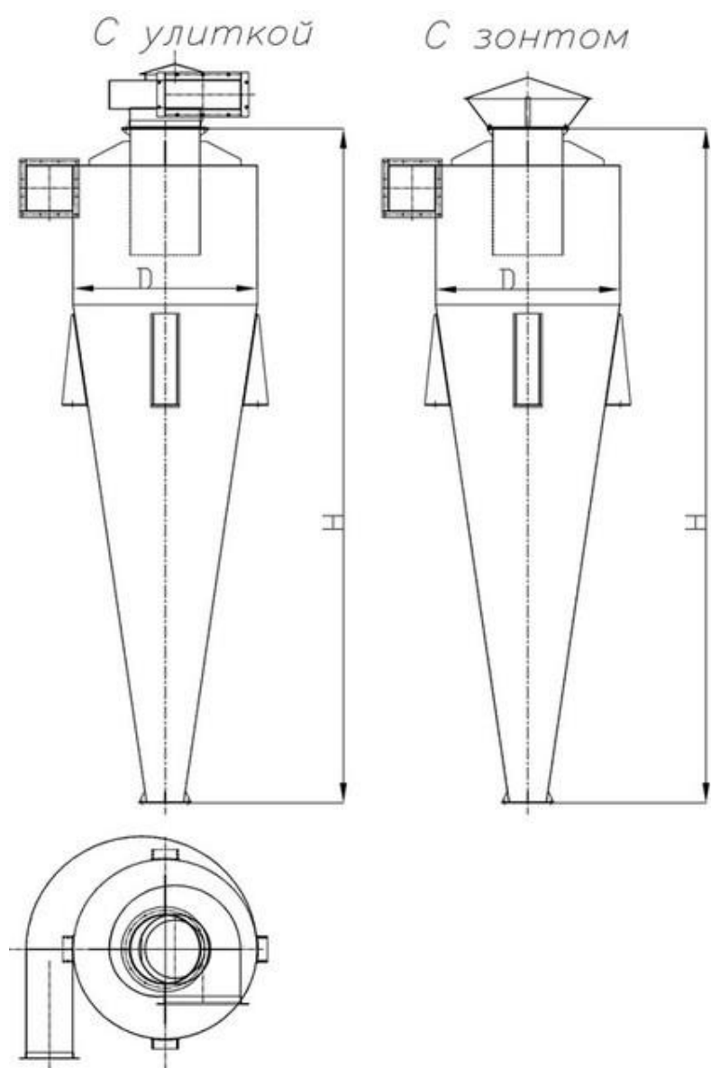
Технические характеристики циклонов УЦ
